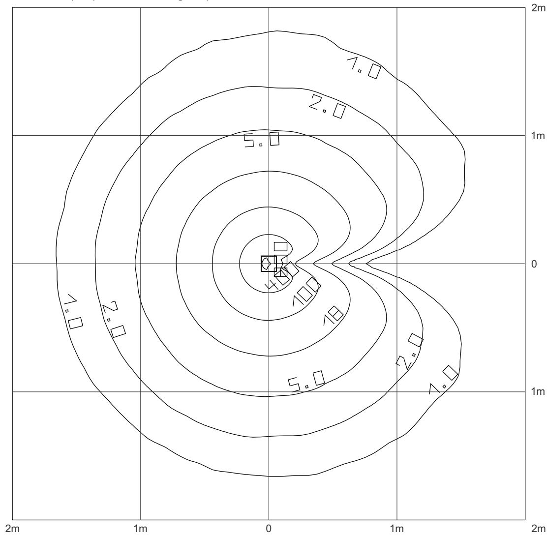
ISOLÍNEA (Lux). Altura del Hongo al piso: 33 cm; utilizando COB a 3000°K.
