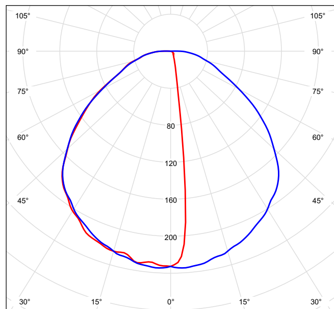
CURVA FOTOMÉTRICA (Cd); utilizando COB a 3000°K.
