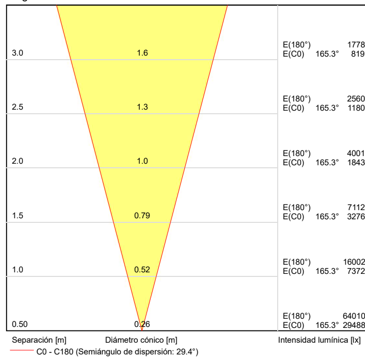
Diagrama Cónico
